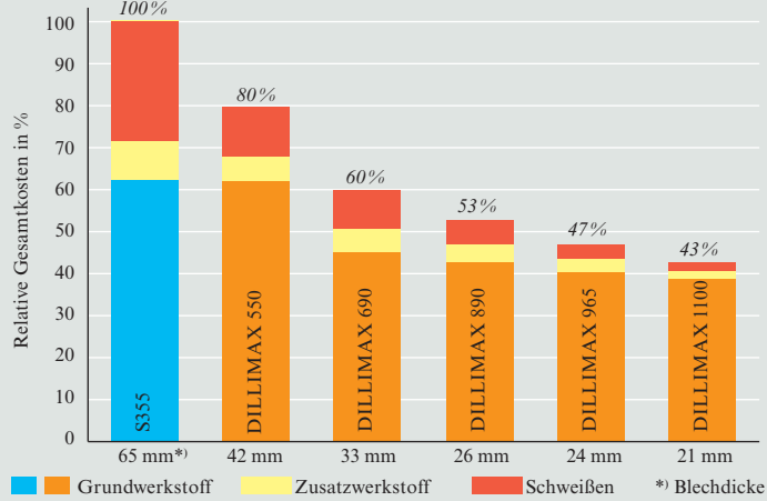
Bild 2: Material- und Verarbeitungskosten: DILLIMAX-Stähle im Vergleich mit konventionellem Stahl S355
